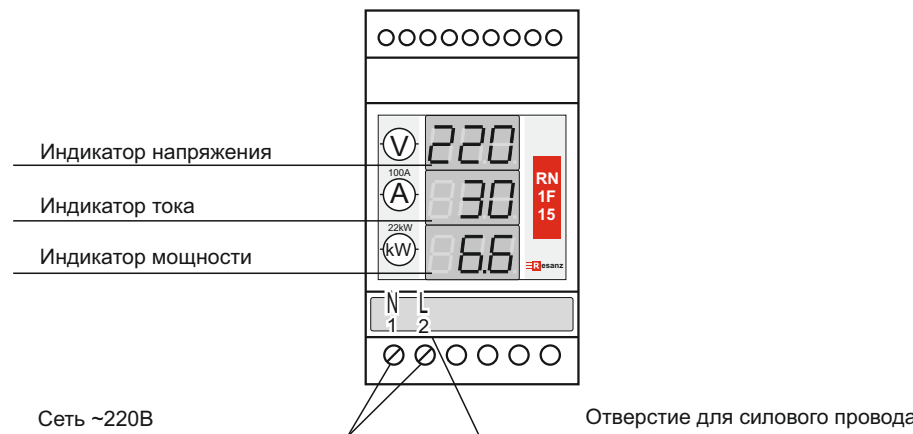
Рис. 1: устройство прибора
