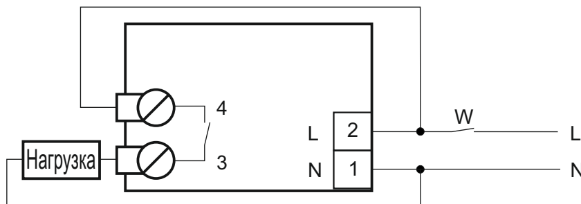
Рис.2. Схема подключения нагрузок к устройству RN 1F-73
