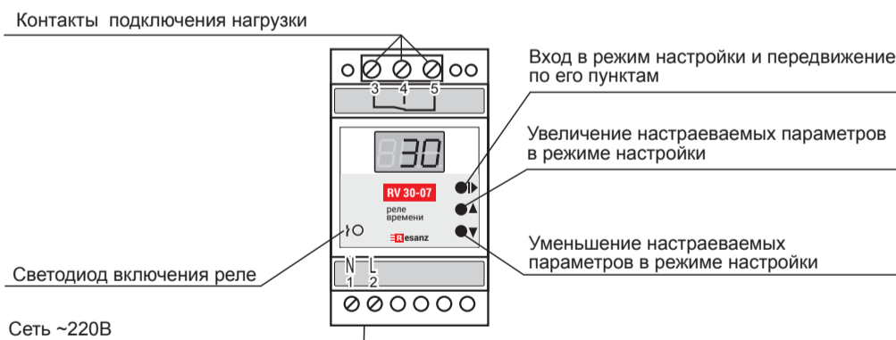
Рис. 1: устройство прибора
